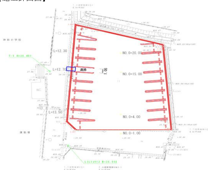
【施工計画図】
