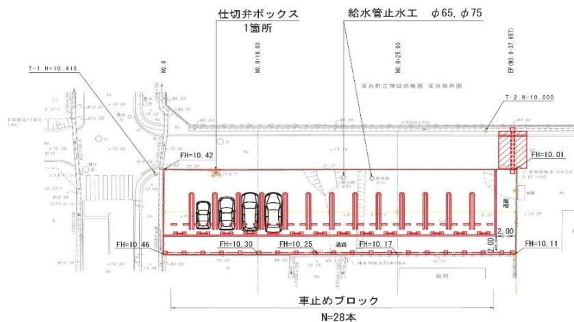
【施工計画図】
